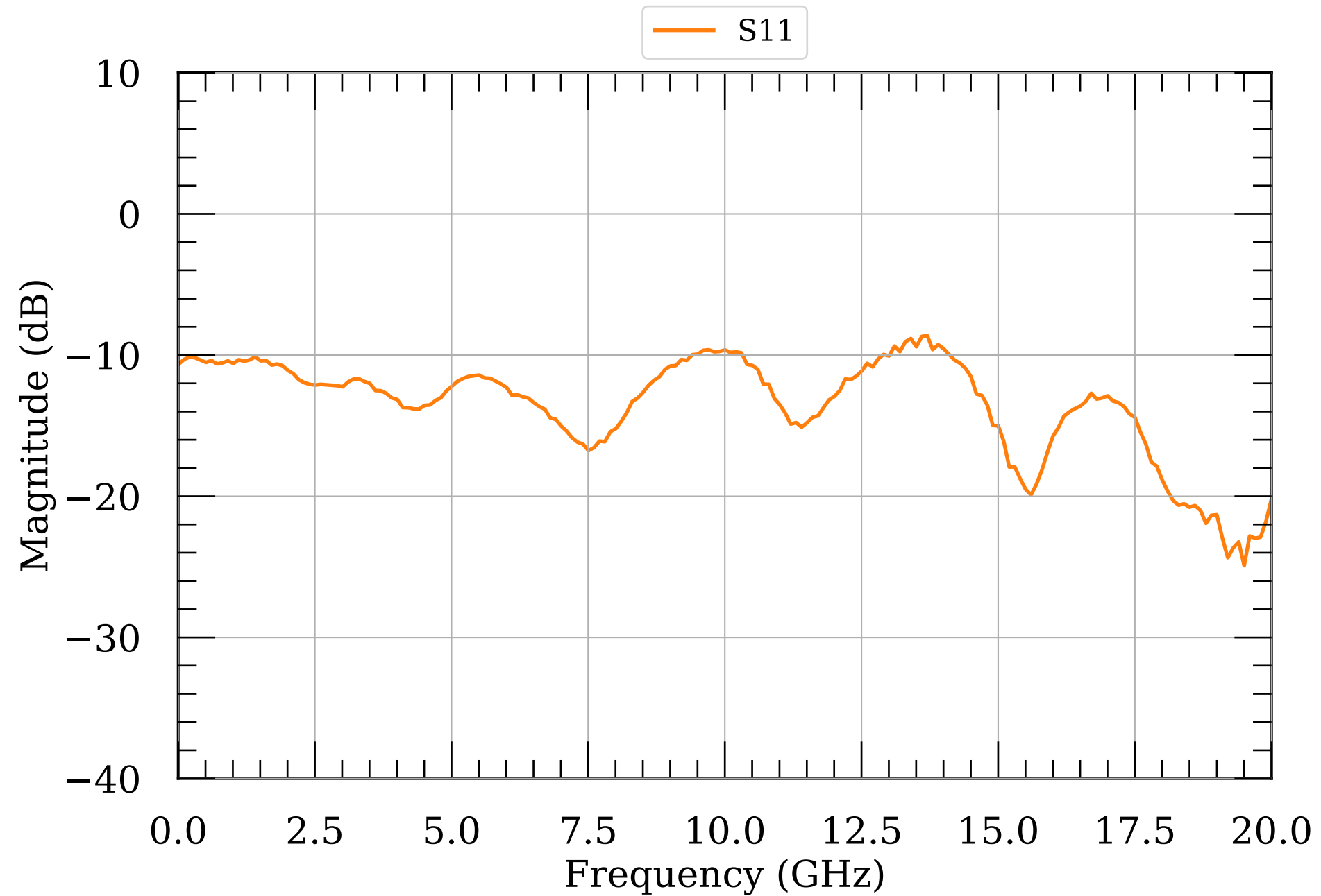
LNA S-params module022v2
